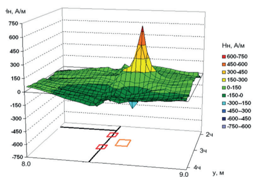
Распределение нормальной составляющей напряженности магнитного поля в локальной зоне сетки трещин и кольцевого сварного шва. □ — обозначена проекция сетки трещин. □ — обозначены проекции дефектов сварного шва. — — обозначены проекции сварных швов.
